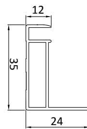
SECTION PROFIL
